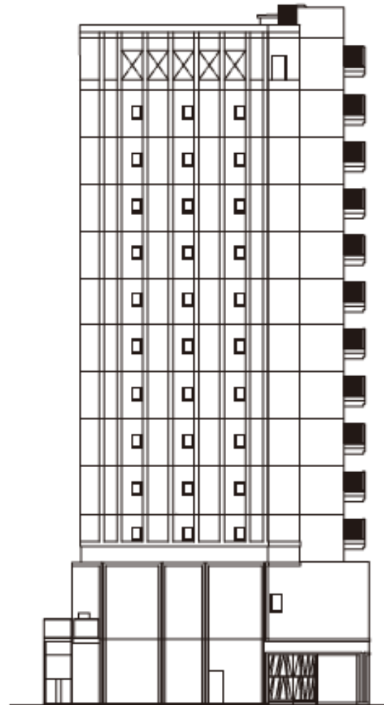
EAST SIDE 【東側立面図】
